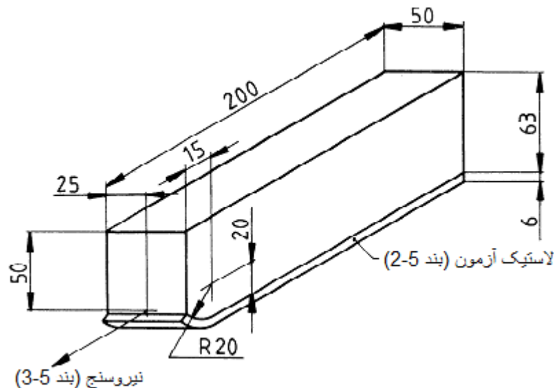
شکل ۱- قطعه آزمون
