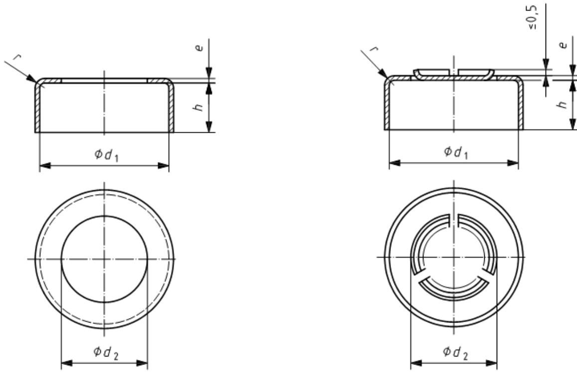
الف) نوع A: درپوش آلومینیومی با سوراخ مرکزی
