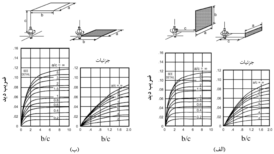
شکل خ-۱. ضرب دید تابشی میان بدن یک شخص نشسته و سطوح مستطیلی اطراف؛ (الف) سطوح عمودی، (ب) سطوح افقی.
